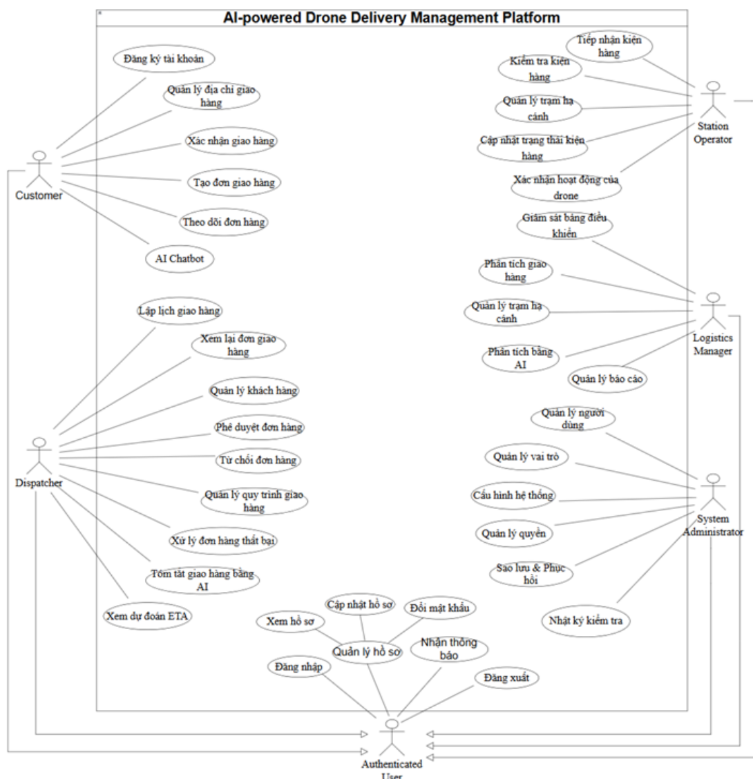
Hình 3.2: Use Case Diagram tổng thể
